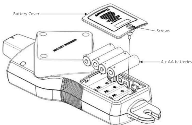
Figura 5.2: Trocando a bateria do receptor
