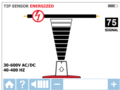
Figure 3.1i Récepteur indiquant le signal détecté en mode CAPTEUR DE POINTE sous tension
