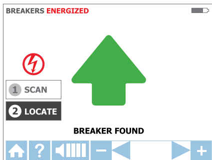
Figura 3.3e Modo de UBICACIÓN; el receptor identificó el interruptor
