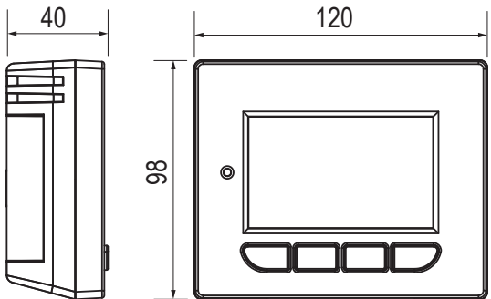
Dimensions pour le montage mural
